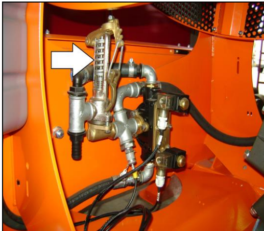
61J. Spoelwaterdrukregelaar
