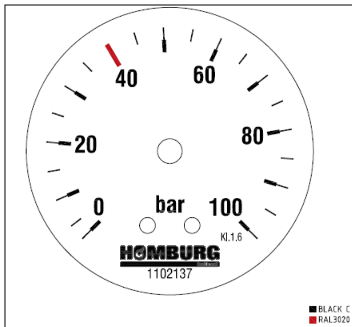
18. Spülwasserdruckmesser
