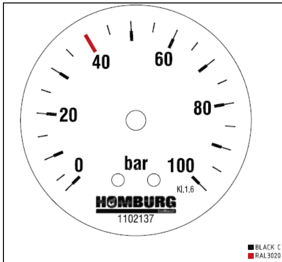
18. Spülwasserdruckmesser
