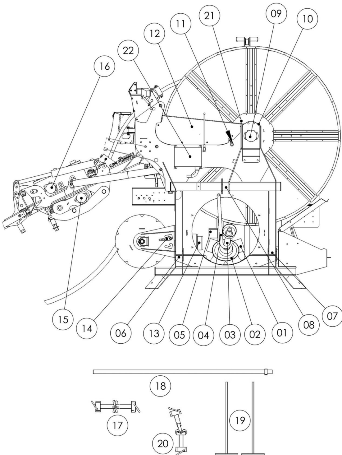
51 Hoofdcomponenten Hurricane voorzijde
